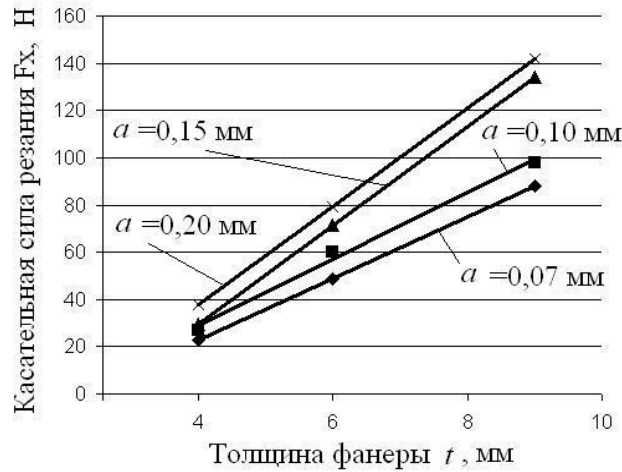
Рис. 3. Зависимость касательной силы резания от толщины фанеры при различных значениях толщины срезаемого слоя a при строгании кромки
