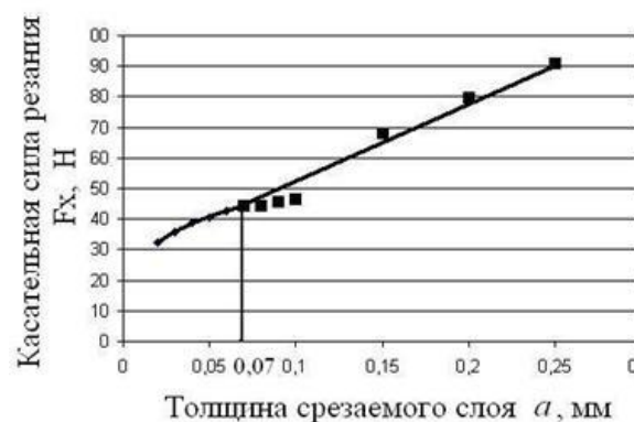
Рис. 2. Зависимость касательной силы резания от толщины срезаемого слоя при строгании поперечных кромок фанеры
