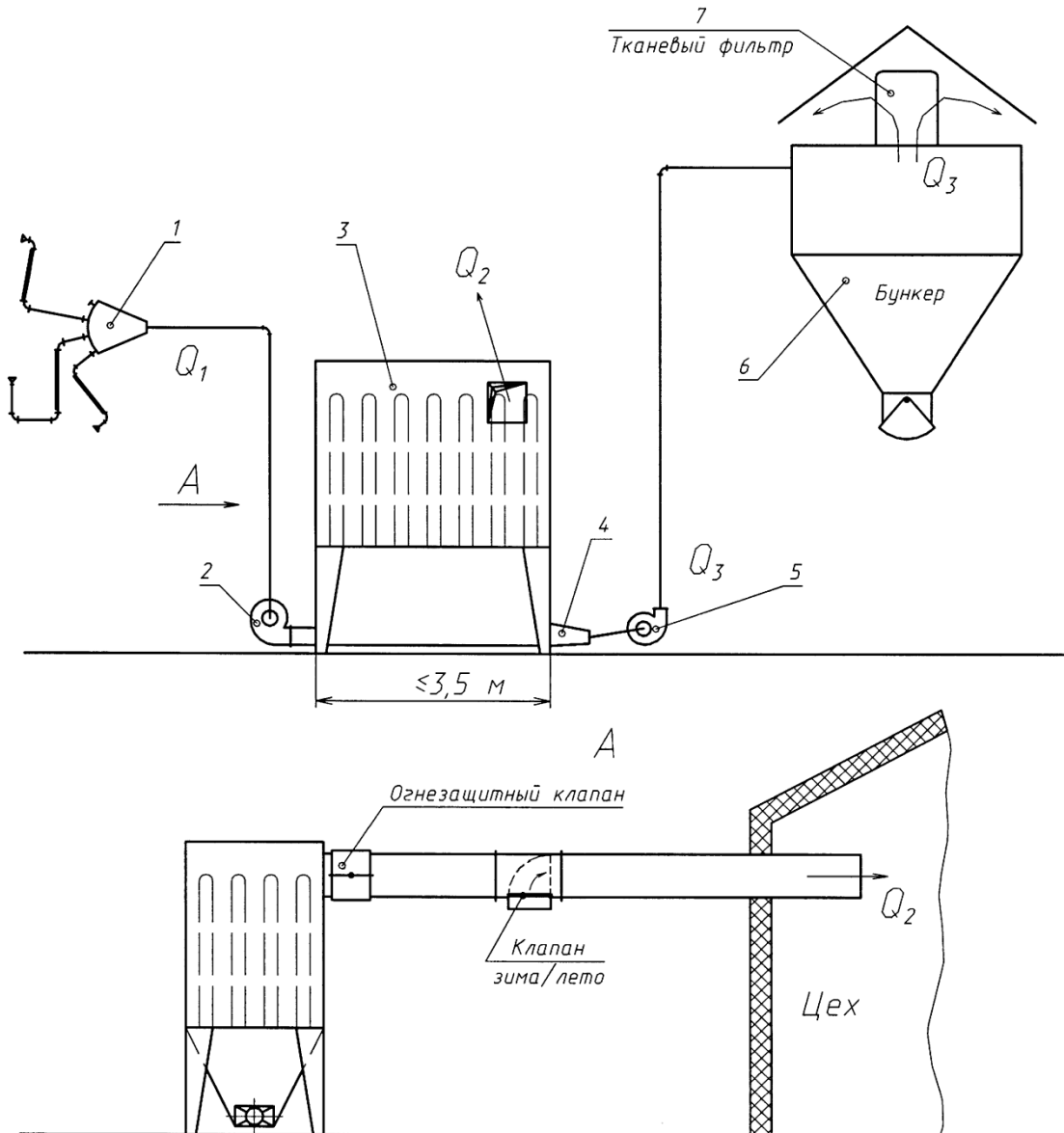
Рисунок – Схема аспирационной системы с упрощенной фильтровальной установкой:
