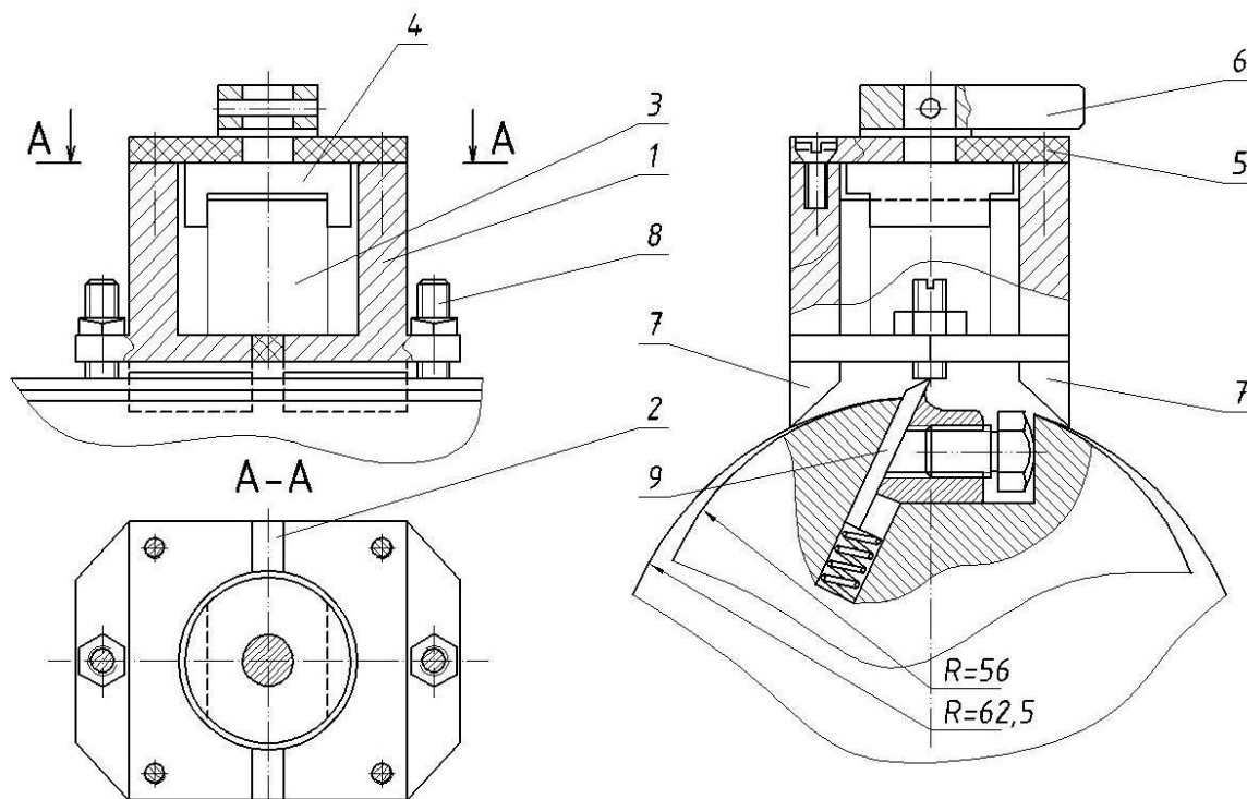
Рисунок – Магнитное устройство для установки ножей в сборных фрезах
