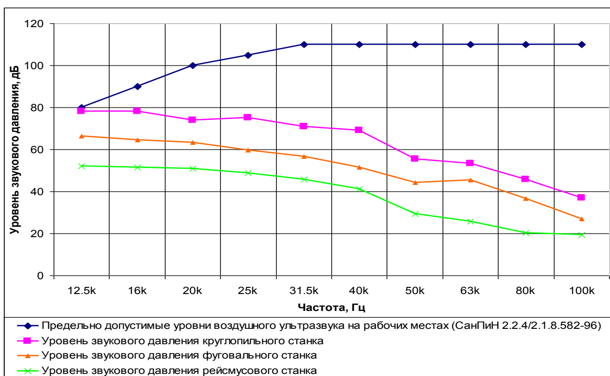
Рис. 1. Результаты измерений уровней воздушного ультразвука на рабочих местах фуговального (СФА3-1), рейсмусового (СР8-4) и круглопильного (Ц5-1А) станков.
