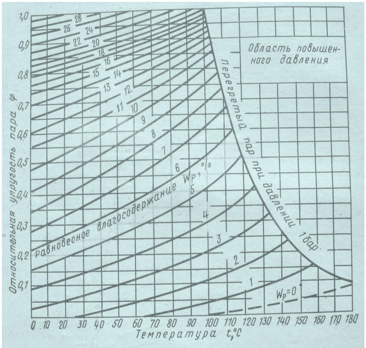
Рис. 1. Исходная диаграмма равновесной влажности древесины.
