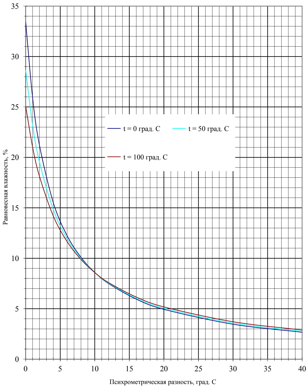
Рис. 2. Диаграмма равновесной влажности древесины, построенная по уравнению 2.
