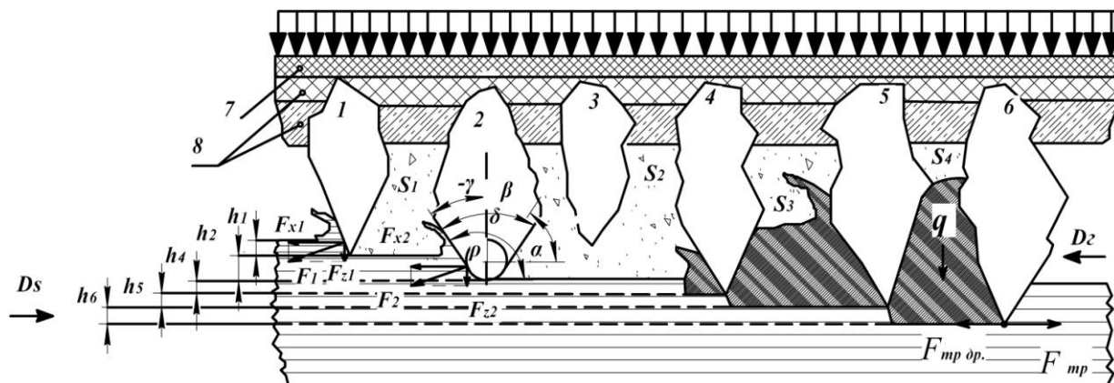
Рисунок 4 - Схема резания абразивным зерном при шлифовании древесины
