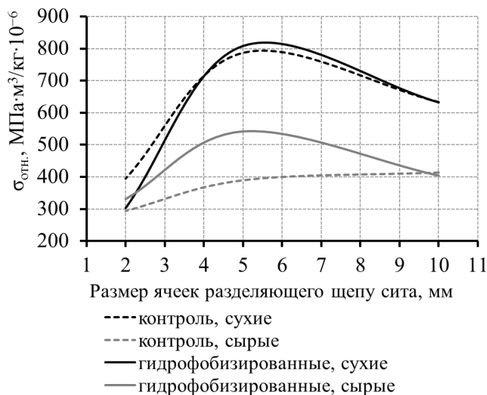
Рис. 2. Прочность арболита на сжатие
