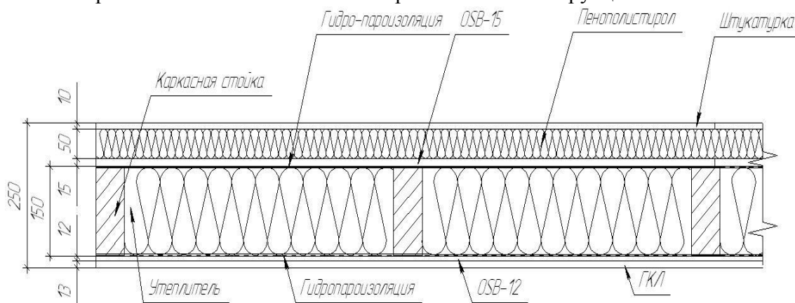
Рисунок 1 – Стеновая панель
