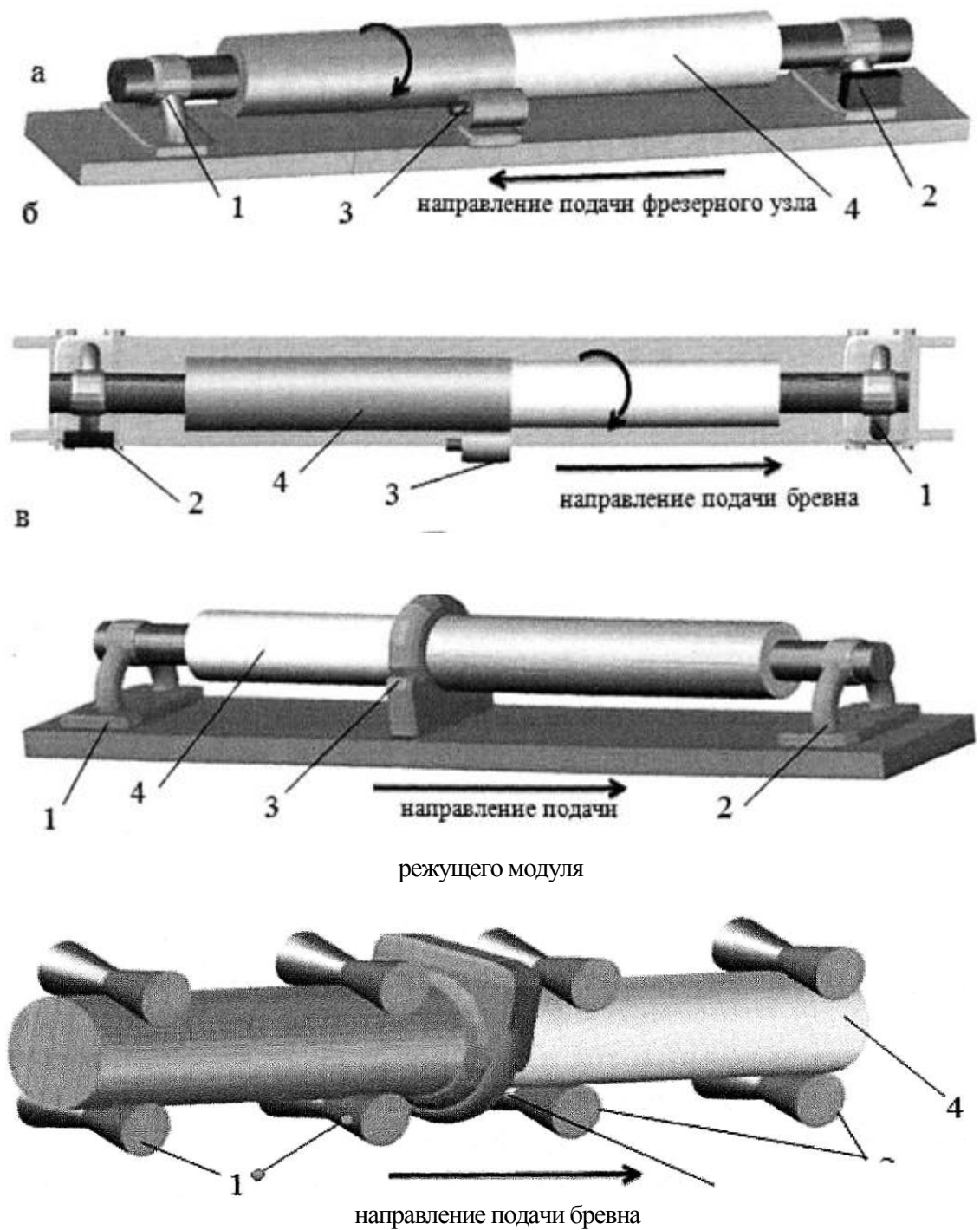
Рис. 1. Принципиальные схемы станков для производства оцилиндрованных деталей строительного назначения. Станки периодического действия: а - центрального типа с вращающимся бревном и подвижным фрезерным узлом: 1 - подвижная зажимная бабка; 2 - зажимная бабка с приводом вращения бревна; 3 - подвижный фрезерный узел; 4 - обрабатываемое бревно; б - центрального типа с надвиганием вращающегося бревна на стационарный фрезерный узел: 1 - подвижная зажимная бабка; 2 - зажимная бабка с приводом вращения бревна; 3 — стационарный фрезерный узел; 4 — обрабатываемое бревно; в — центрального типа с неподвижным бревном: 1, 2 — зажимные бабки; 2 - подвижной режущий модуль; 4 - обрабатываемое бревно. Станки проходного типа: г — 1 — подающие вальцы; 2 — приемные вальцы; 3 - стационарный режущий модуль; 4 - обрабатываемое бревно
